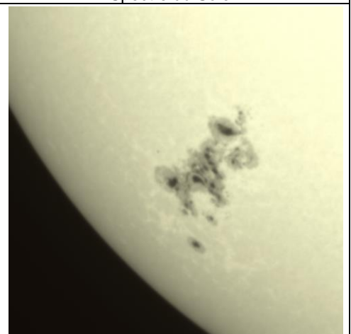
Taches solaires
