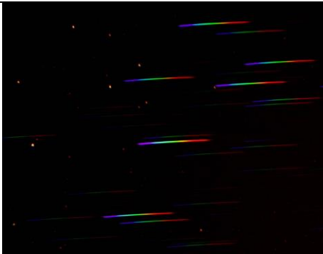
Spectres des étoiles des Pléiades-M45
